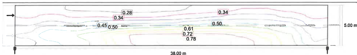
Observator 2: Valoarea de întreținere, densitatea luminii cu carosabil uscat [ \text{cd/m}^2 ] (Linii Isolux)
