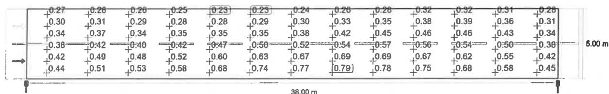
Observator 1: Valoarea de întreținere, densitatea luminii cu carosabil uscat [ \text{cd/m}^2 ] (Raster valoric)
