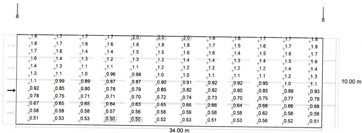
Observator 2: Densitatea luminii la instalația nouă [cd/m²] (Raster valoric)
