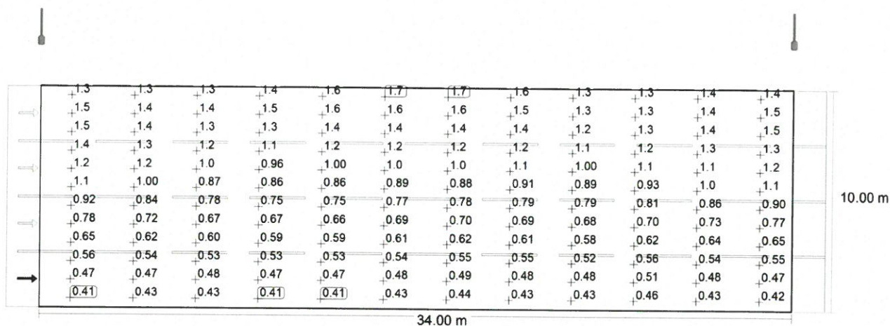
Observator 1: Valoarea de întreținere, densitatea luminii cu carosabil uscat [cd/m 2 ] (Raster valoric)
