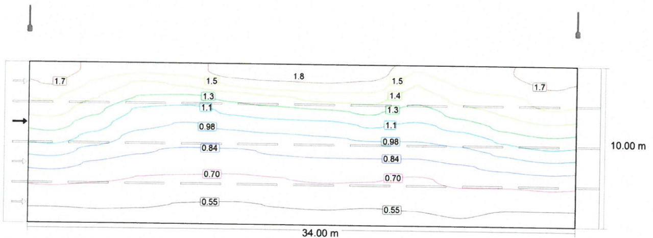
Observator 3: Densitatea luminii la instalația nouă [cd/m 2 ] (Linii Isolux)
