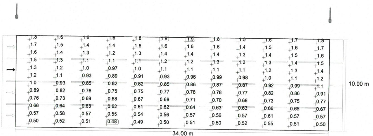
Observator 3: Densitatea luminii la instalația nouă [cd/m 2 ] (Raster valoric)
