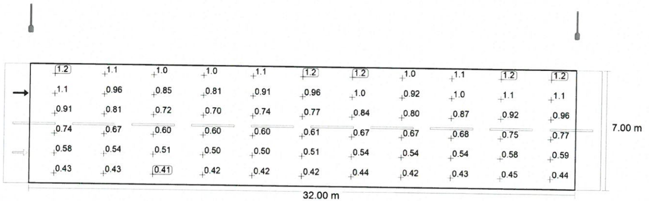
Observator 2: Valoarea de întreținere, densitatea luminii cu carosabil uscat [ \text{cd}/\text{m}^2 ] (Raster valoric)
