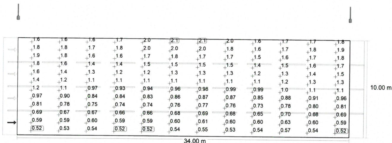
Observator 1: Densitatea luminii la instalația nouă [cd/m 2 ] (Raster valoric)
