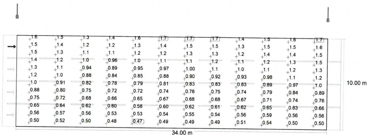
Observator 4: Densitatea luminii la instalația nouă [cd/m 2 ] (Raster valoric)
