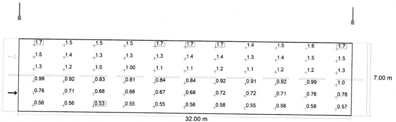
Observator 1: Densitatea luminii la instalația nouă [cd/m 2 ] (Raster valoric)
