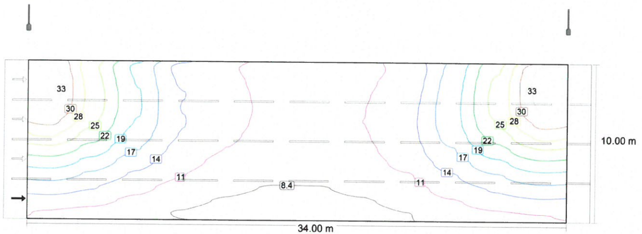
Valoarea de întreținere, intensitatea de iluminare orizontală [lx] (Linii Isolux)
