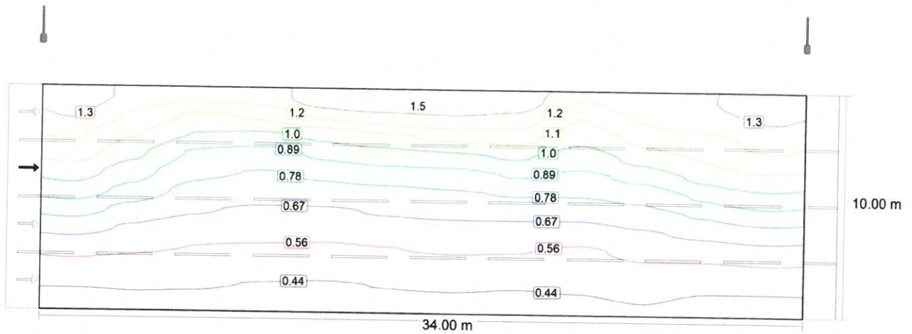
Observator 3: Valoarea de întreținere, densitatea luminii cu carosabil uscat [\text{cd/m}^2] (Linii Isolux)
