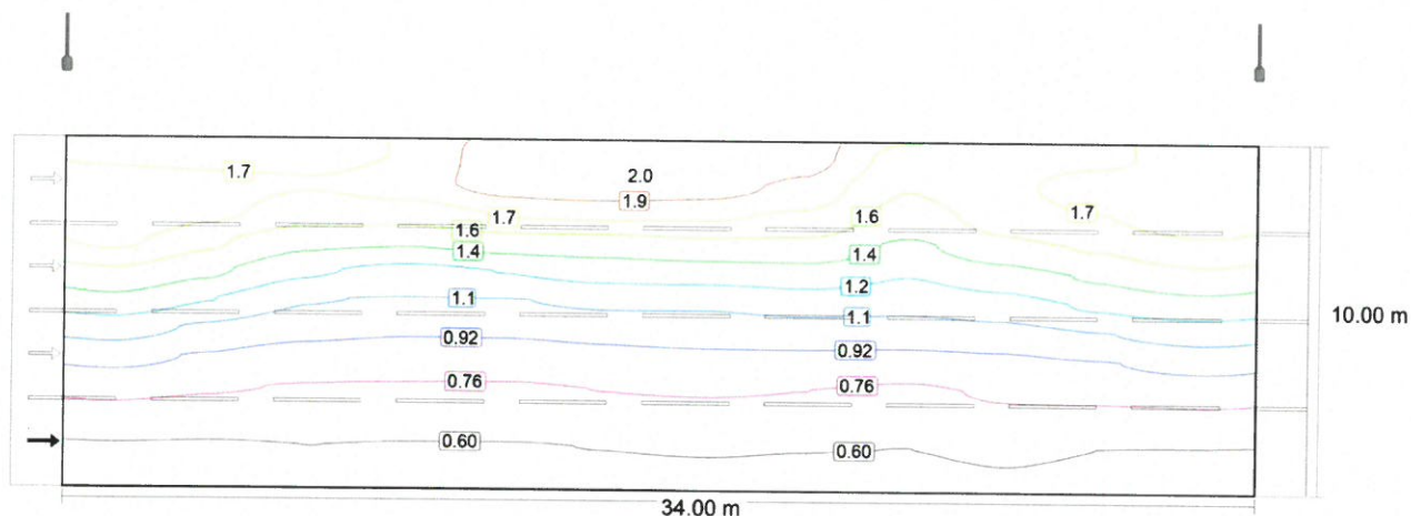
Observator 1: Densitatea luminii la instalația nouă [cd/m 2 ] (Linii Isolux)
