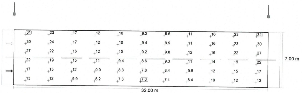
Valoarea de întreținere, intensitatea de iluminare orizontală [lx] (Raster valoric)
