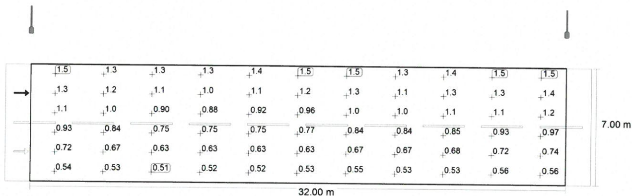
Observator 2: Densitatea luminii la instalația nouă [cd/m 2 ] (Raster valoric)
