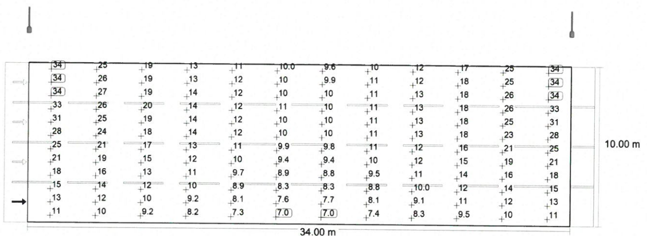
Valoarea de întreținere, intensitatea de iluminare orizontală [lx] (Raster valoric)
