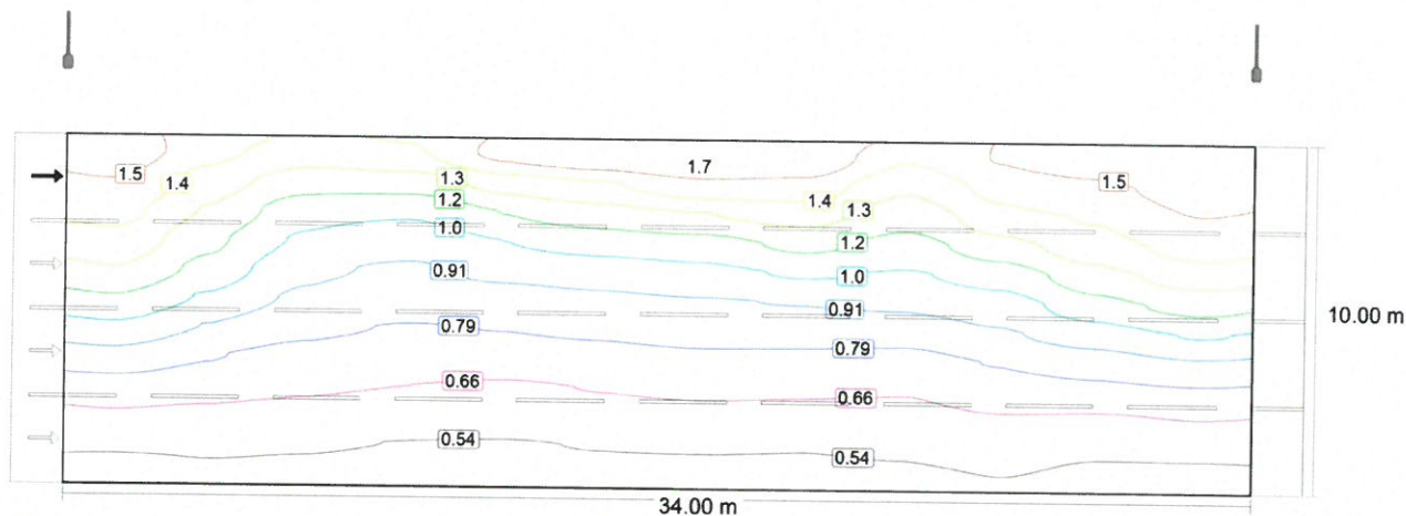
Observator 4: Densitatea luminii la instalația nouă [cd/m 2 ] (Linii Isolux)
