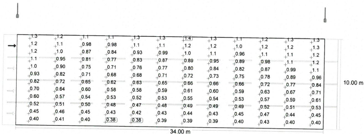
Observator 4: Valoarea de întreținere, densitatea luminii cu carosabil uscat [cd/m 2 ] (Raster valoric)
