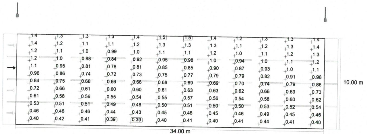
Observator 3: Valoarea de întreținere, densitatea luminii cu carosabil uscat [\text{cd/m}^2] (Raster valoric)
