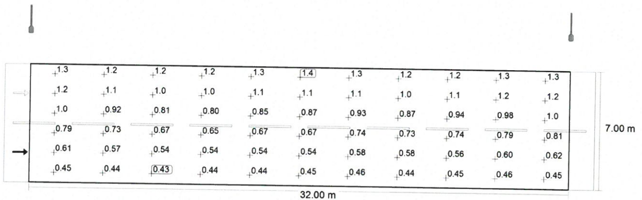
Observator 1: Valoarea de întreținere, densitatea luminii cu carosabil uscat [ \text{cd}/\text{m}^2 ] (Raster valoric)
